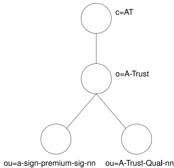
Abbildung 2: a.trust Verzeichnisbaum
